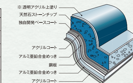
断面構成図
