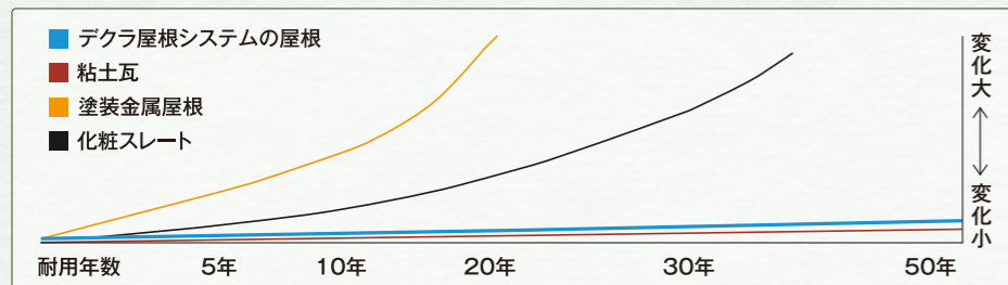
デクラ屋根システムの経年変化
