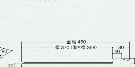
本体断面形状(単位mm)
